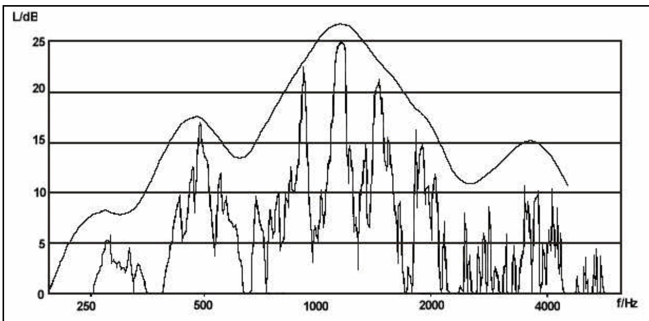
Abb. 6: Frequenzkurve einer Fabrikvioline mit überlagertem Glättungskurve
