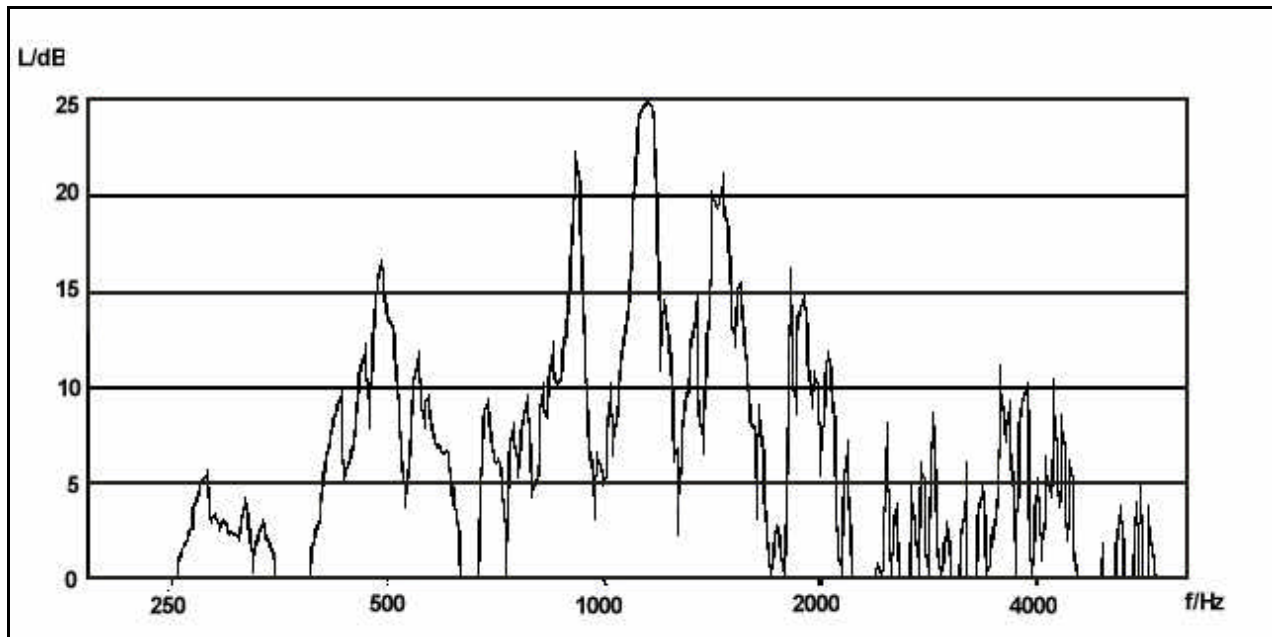
Abb. 1b) Frequenzkurve einer Fabrikvioline
