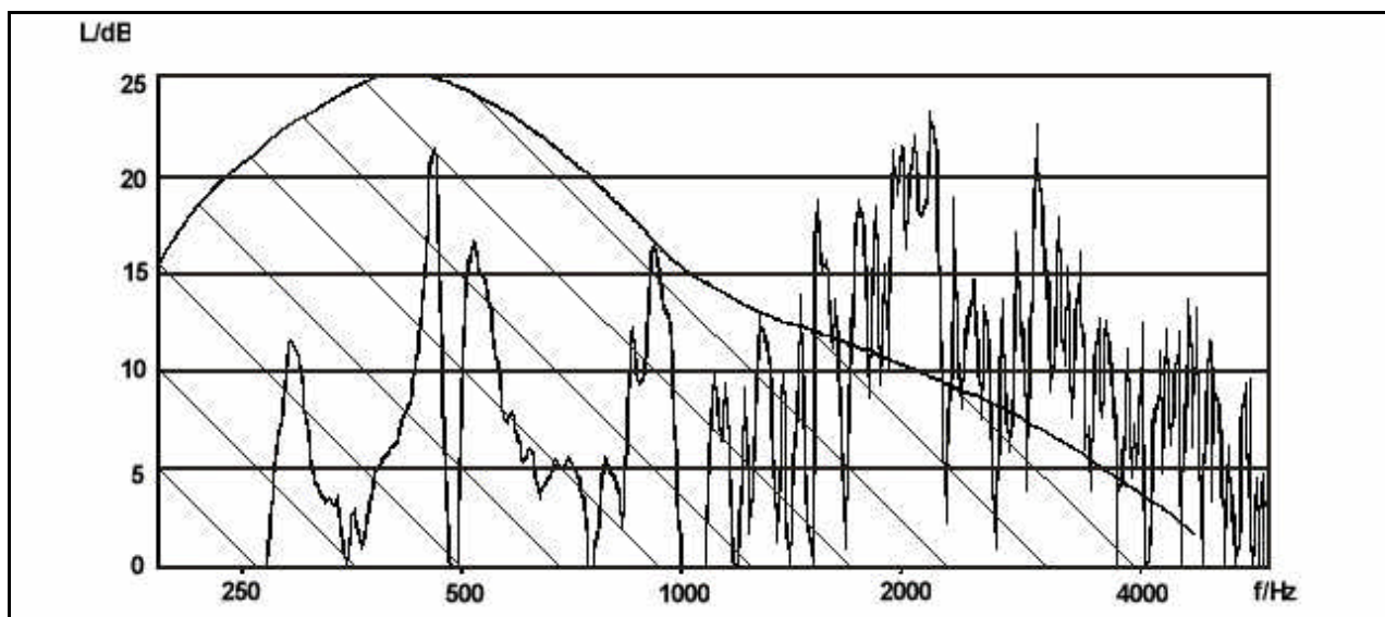
Abb. 4: Durchschnittsspektrum des Orchesters, berlagert mit der Frequenzkurve von Abb. 1a (P. Guarneri 1742). Nach Greiner 1992.
