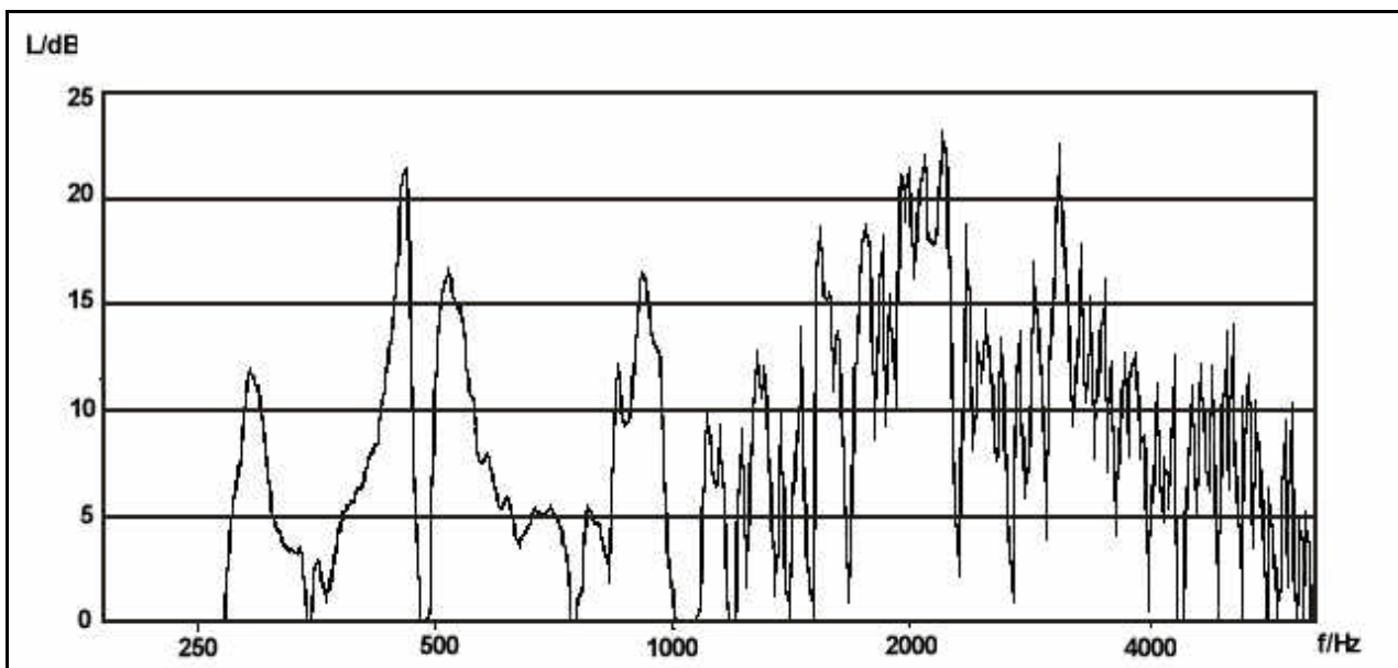
Abb. 1a) Frequenzkurve einer P. Guarnerius von 1742
