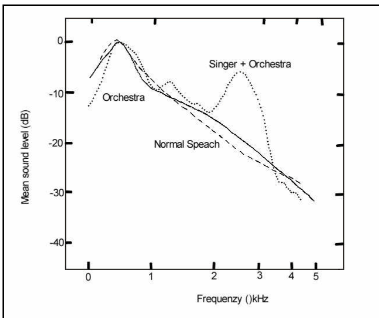
Abb. 3: Langzeitspektren von a) Orchesterklang (ausgezogene Kurve); b) Gesangssolist (punktierter Kurve), c) gesprochener Sprache (gestrichelte Kurve). Aus SUNDBERG (1987, S. 123).
