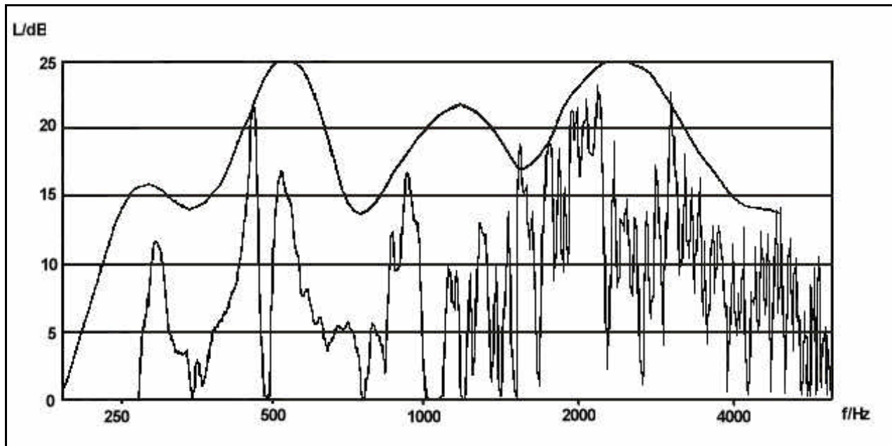
Abb. 7: Frequenzkurve einer Guarnerius-Violine mit überlagerter Glättungskurve einer Amati (Abb. 5).
